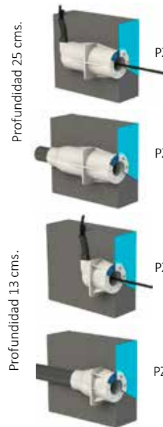
ESQUEMA DE INSTALACION Sistema PressFit™
