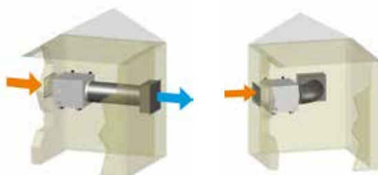
INSTALACIÓN CON EXTRACCIÓN DE AIRE MURAL
