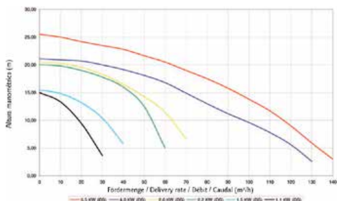
BOMBAS TRIFÁSICAS
