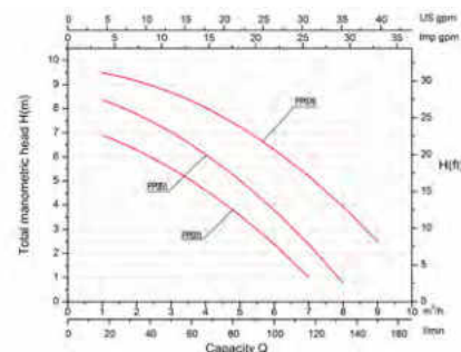
Curvas de rendimiento hidráulico Hydraulic paraformance curves Courbes de performances hydrauliques Curve delle prestazioni idrauliche
