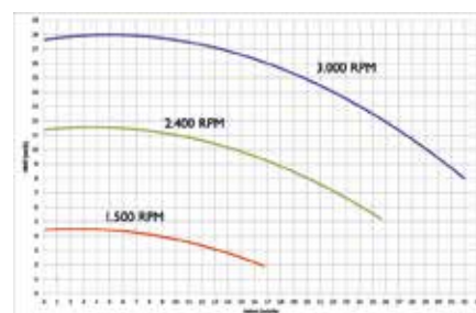
Tristar VSTD 2,0 CV/HP
