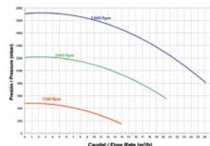
Tristar VSTD 1,5 CV/HP
