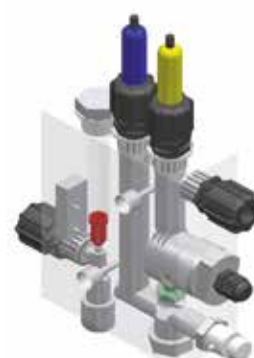
Célula de cloro amperométrica PRO-CG-CL3. Escala de medición 0-5 ppm; Cuerpo plexiglass, sensor de flujo, electrodo cobre/platino. No incluida en la HDE TOP CL. Chlorine amperometric cell PRO-CG-CL3. Measurement range 0-5 ppm; Plexiglass body, flow sensor, electrode copper / platinum. Not included in HDE TOP CL.
